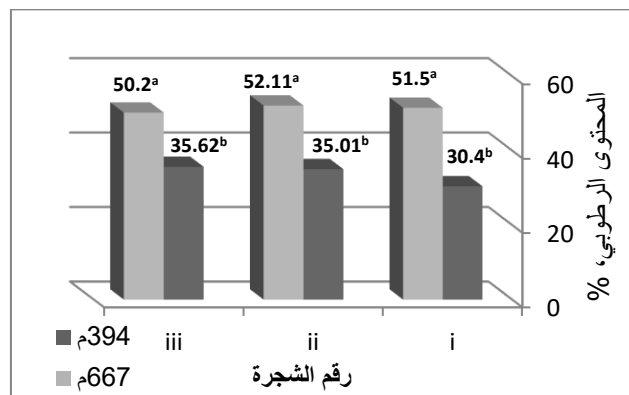
شكل 1: متوسط قيم المحتوى الرطوبي % في خشب الشماري في موقعي الدراسة.
